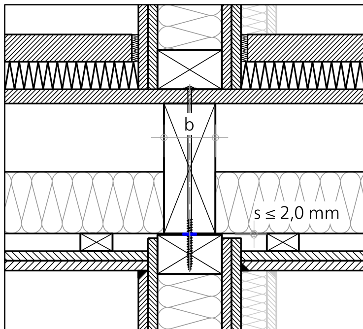
Abbildung 8: Trennwand-Deckenanschlüsse Holztafelbau mit Spaltmaß s \leq 2,0 mm
