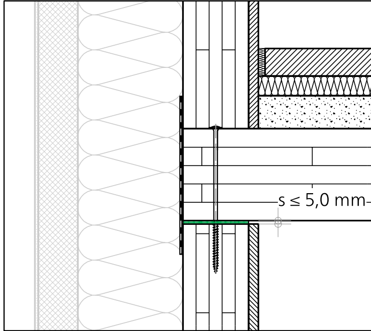
Abbildung 20: Außenwand-Deckenanschluss Massivholzbau mit Spaltmaß s ≤ 5,0 mm
