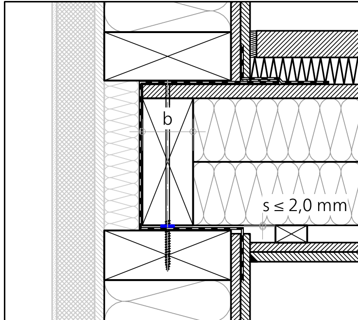
Abbildung 7: Außenwand-Deckenanschlüsse Holztafelbau mit Spaltmaß s \leq 2,0 mm
