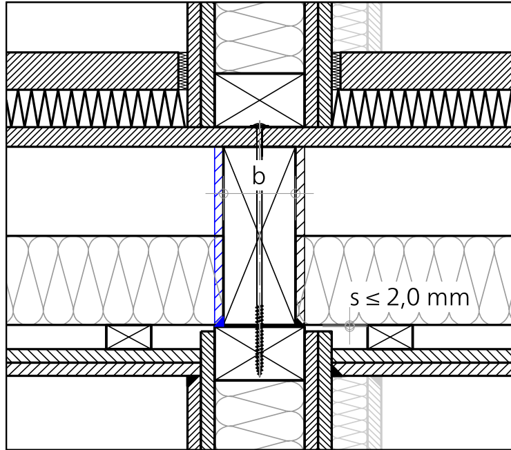
Abbildung 9: Trennwand-Deckenanschluss Holztafelbau mit Spaltmaß s \leq 2,0 mm
