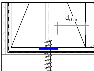
Abbildung 7: Außenwand-Deckenanschlüsse Holztafelbau mit Spaltmaß s \leq 2,0 mm
